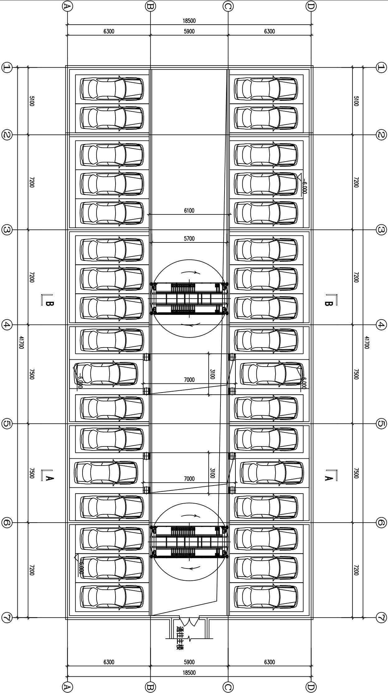
车库负一层平面图
