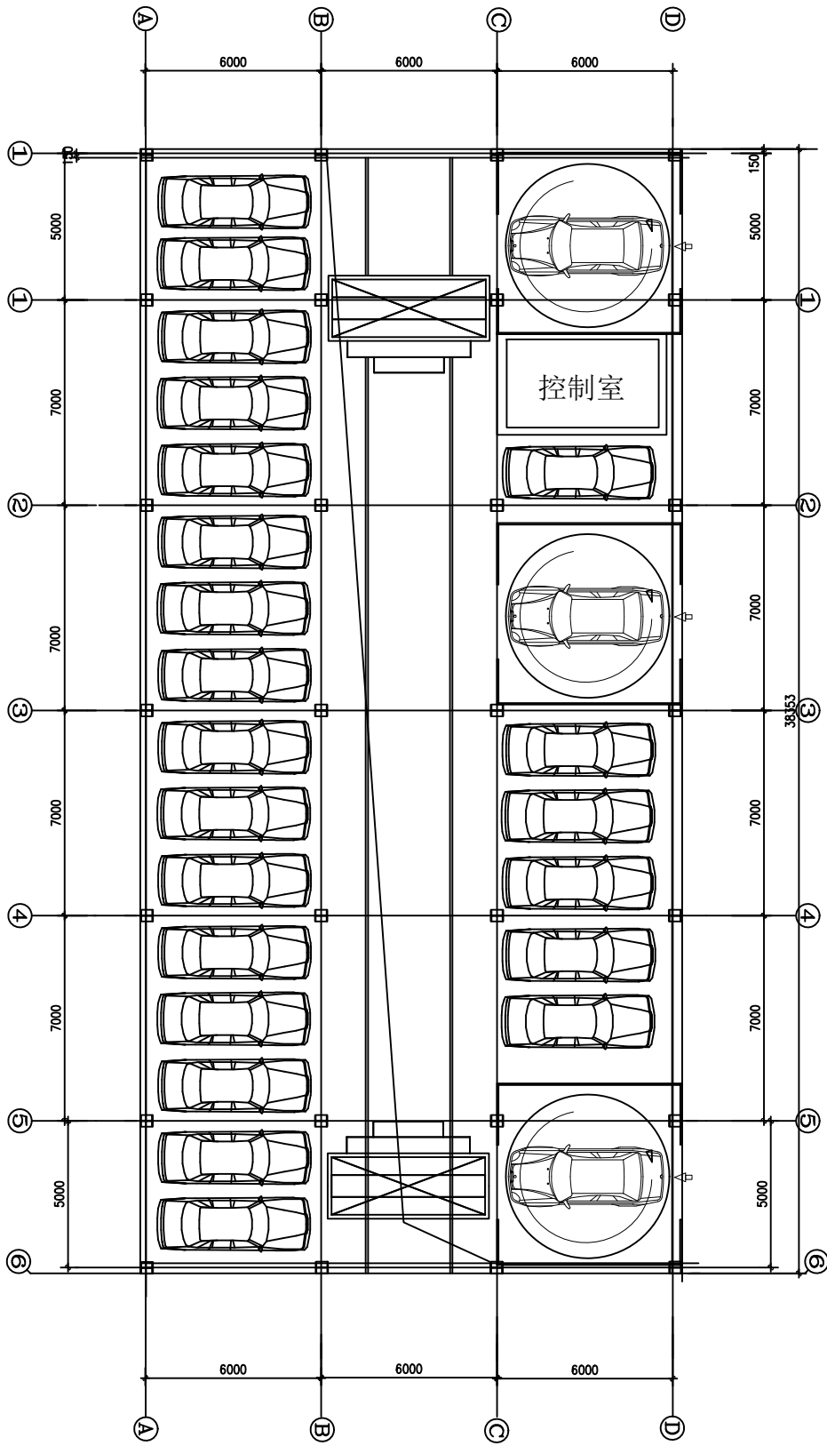
一层平面图 1:100
